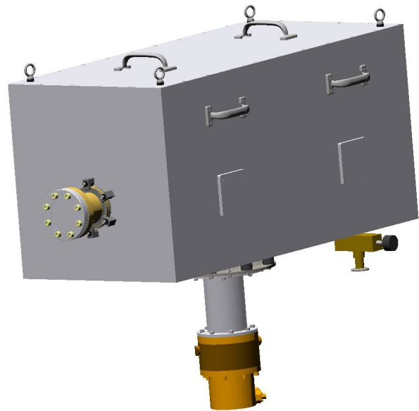
Modelo 3D del criostato de GRANCAIN.
