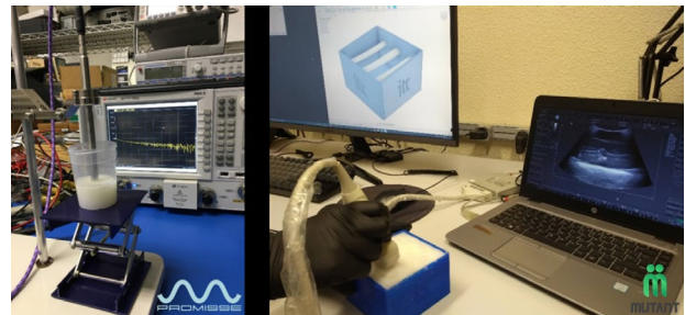
Figura 3: Caracterización experimental de algunos de los fantasmas fabricados en las modalidades de microondas (izquierda) y ultrasonido (derecha).
