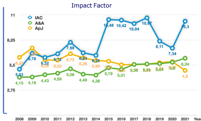
Figura 1: Factor de Impacto de las publicaciones del IAC comparado con las revistas Astronomy and Astrophysics (A&A) y Astrophysical Journal (ApJ)
